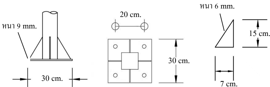
รูปขยายแผ่นเหล็กฐานเสา (Plate) และคียบ
