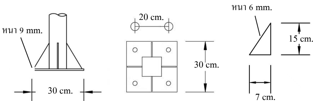
รูปขยายแผ่นเหล็กฐานเสา (Plate) และคريب
